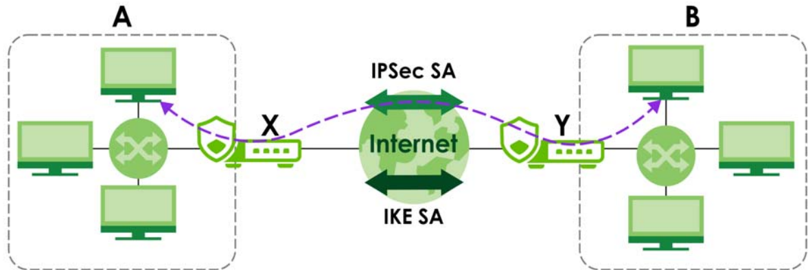
Figure 142 VPN: IKE SA and IPsec SA
